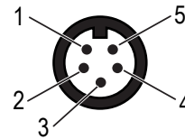
5-pin Mini male pinout
