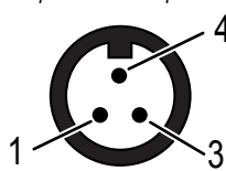
3-pin Mini male pinout
