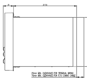
RIGHT/RECHTS
