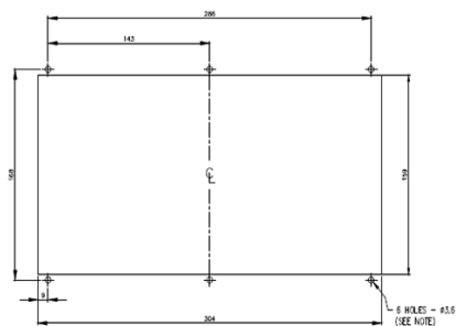
PANEL CUT-OUT/SCHALTAFELAUSSCHNITT
