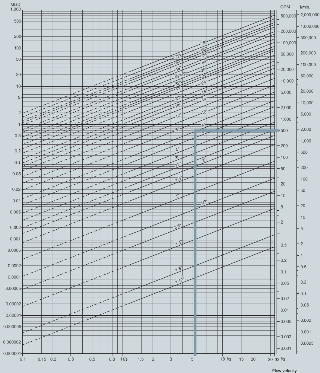
Sizing table ( 1/12'' ... 78'')
