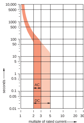
S204UP-Z, 4 pole
