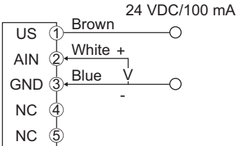
Analog input (V)
