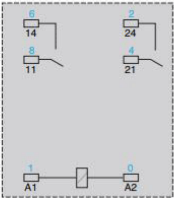
DPST-NO (2 NO):
