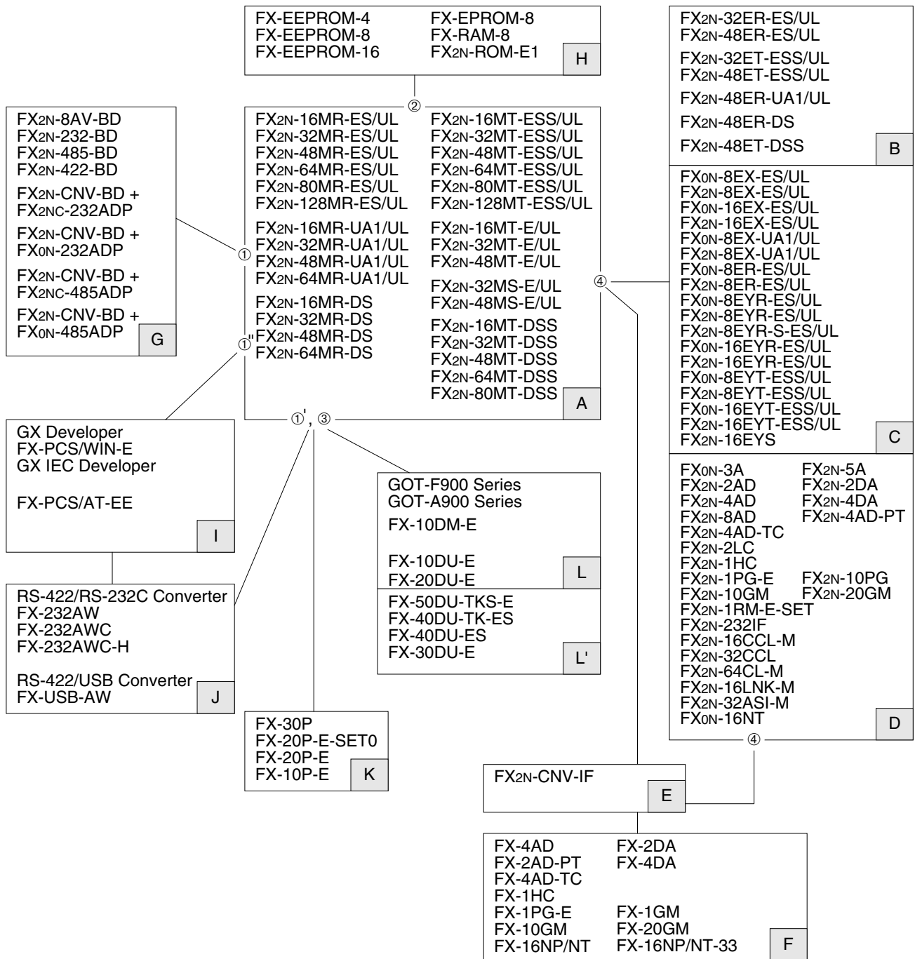
Figure 1.6: ENG ≡ Schematic system FRE ≡ Représentation schématique de la construction du système GER ≡ Schematischer Systemaufbau ITL ≡ Struttura schematica del sistema ESP ≡ Configuración esquemática del sistema
