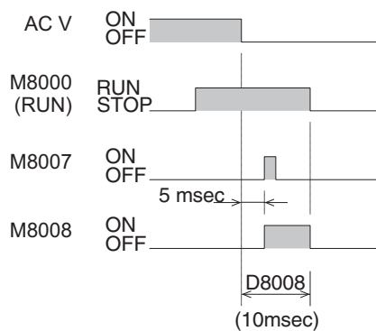
Figure 7.2: ENG ≡ Power down and its associated flags FRE ≡ Indicateurs d'erreurs pour pannes de tension GER ≡ Fehlermerker für Spannungsausfall ITL ≡ Merker di errore per caduta di tensione ESP ≡ Marcadores de fallos/errores para fallo de tensión
