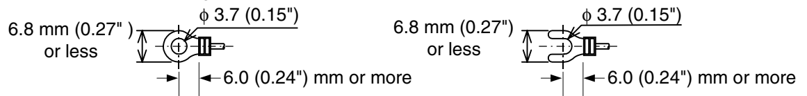
Figure 4.4: ENG ☞ Crimp Terminals for M3.5 Screws FRE ☞ Cosse de câble avec raccordement serti pour vis M3,5 GER ☞ Kabelschuhe mit Quetschanschluss für M3,5-Schrauben ITL ☞ Capocorda con collegamento a scatto per viti M3,5 ESP ☞ Manguitos de cable con conexión de apriete para tornillos M3,5
