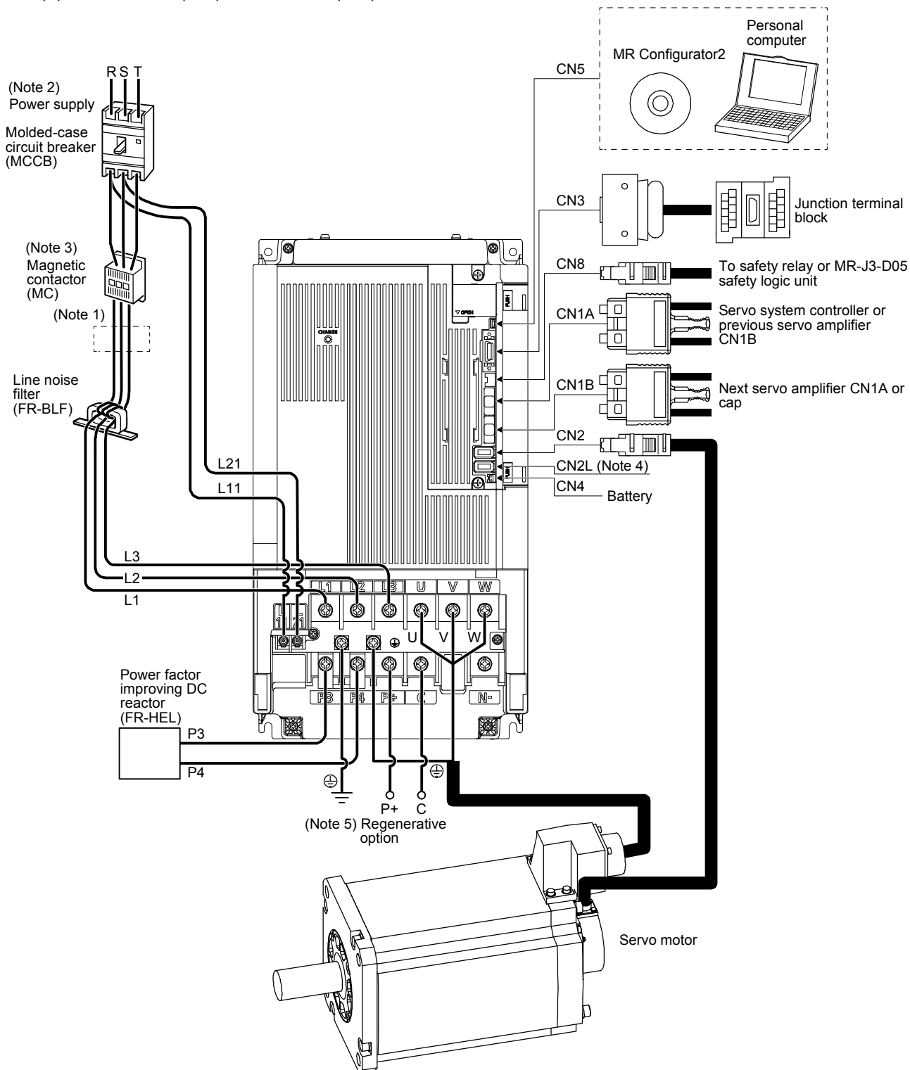
(e) MR-J4-11KB(-RJ)/MR-J4-15KB(-RJ)
