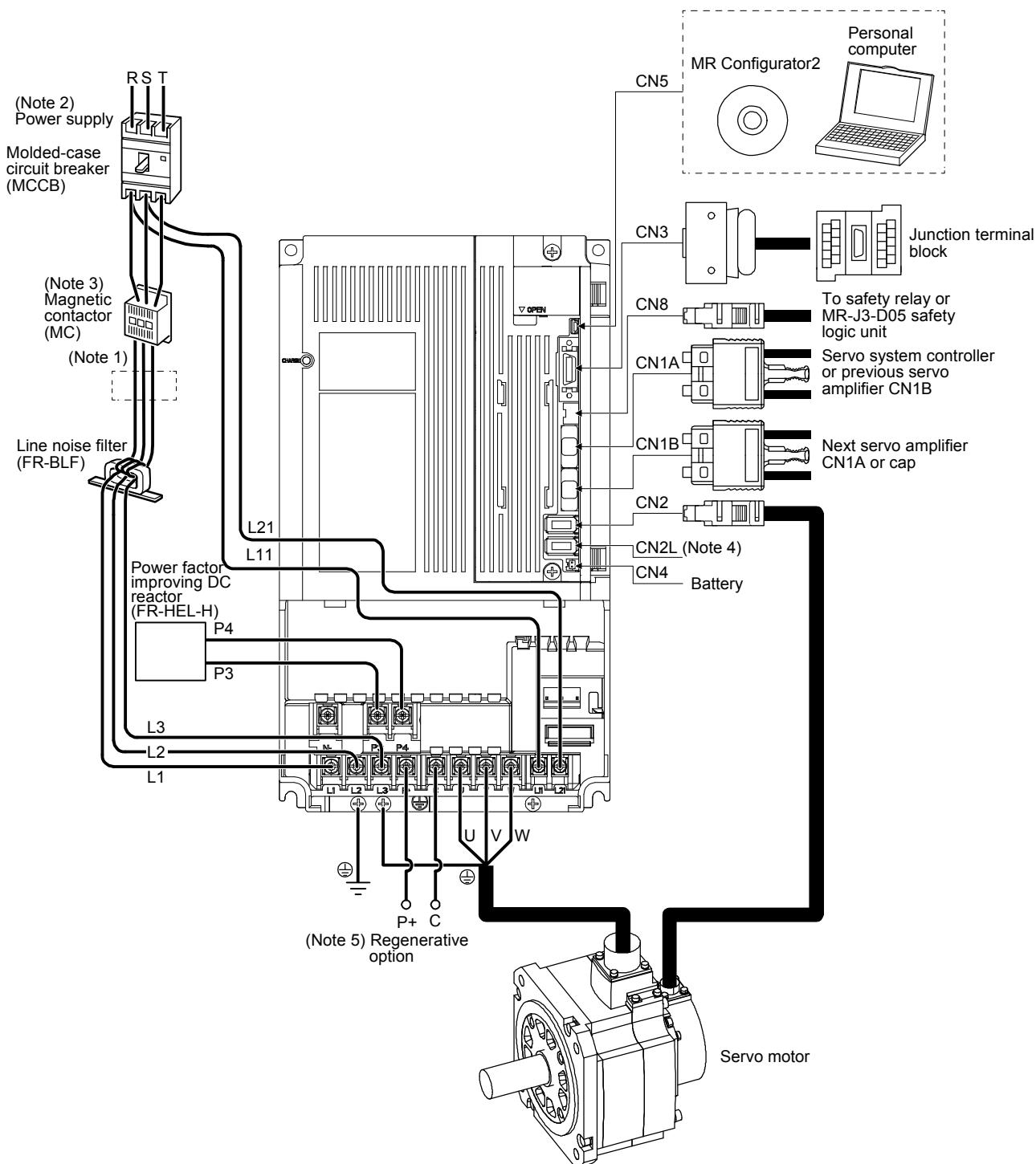
(d) MR-J4-700B4(-RJ)
